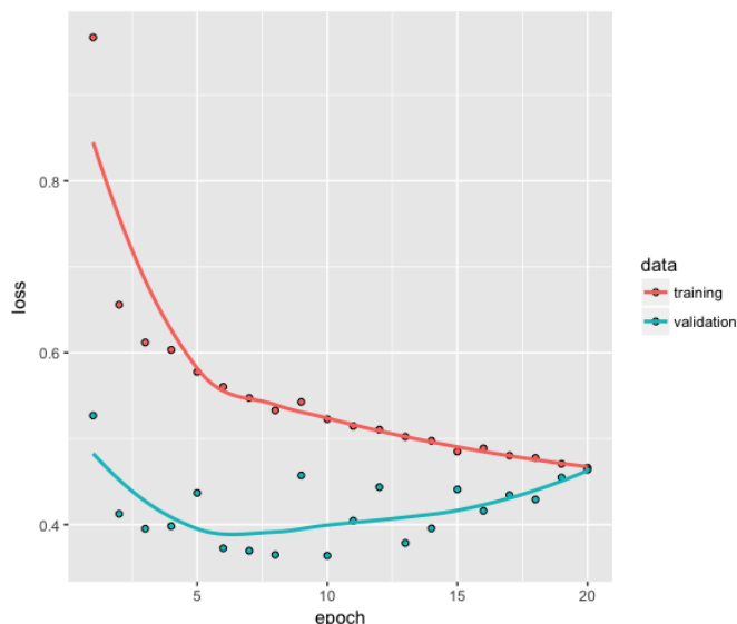
Figure 4. Loss functions de la primera arquitectura en regiones de similar comportamiento.
