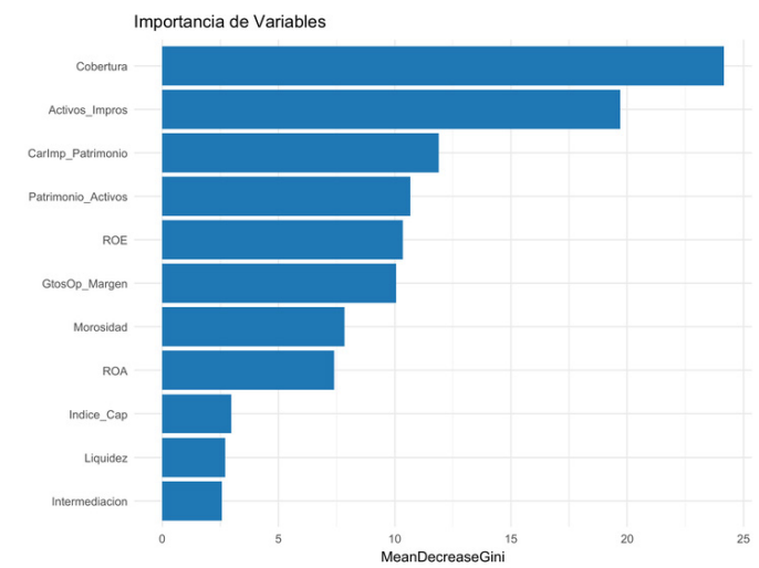
Figura 1. Importancia de variables del modelo Random Forest (Mean Decrease in Gini).
